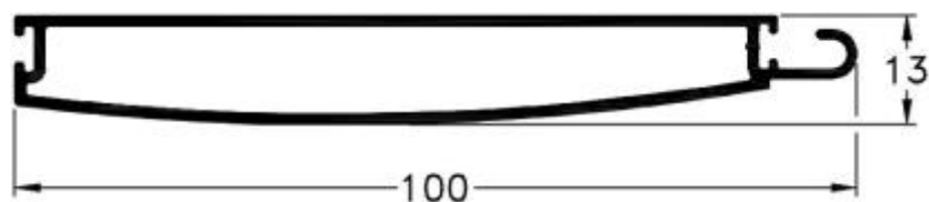
624 - Zócalo Cortina Común Largo std.: 6150 mm peso: 0,76 Kg/m
